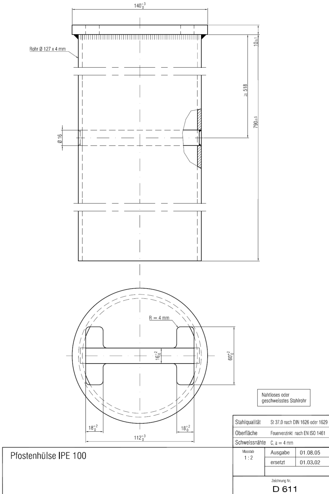
Abb. 2.11 Pfostenhülse IPE 100.
