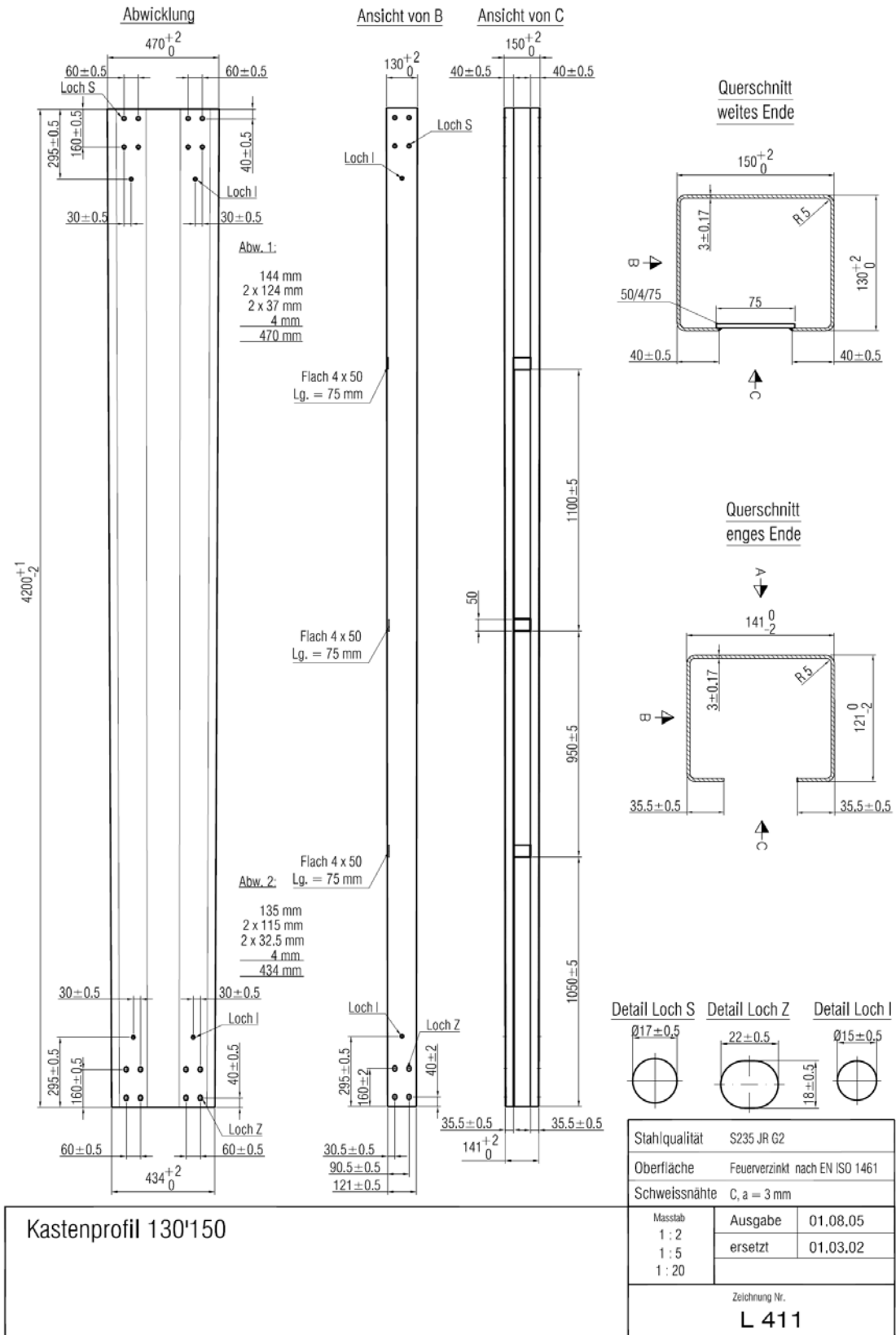
Abb. 2.9 Kastenprofil 130'150.
