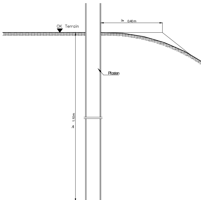
Abb. 4.3 Pfosten gerammt.
