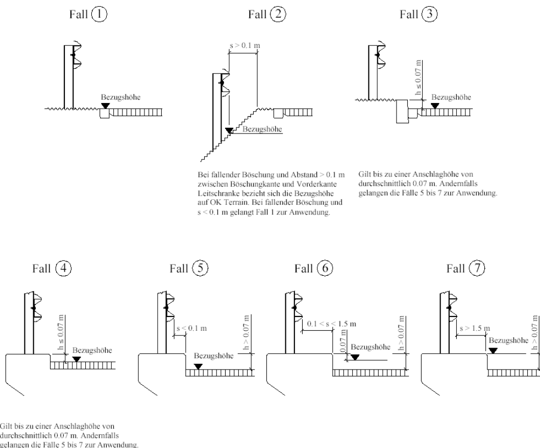
Abb. 6.10 Einbauhöhen.
